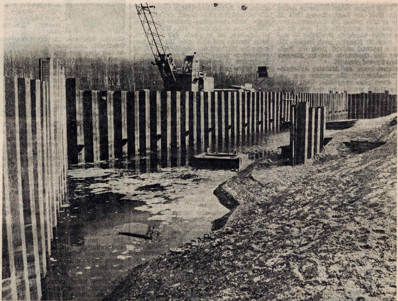
Spundwände wurden in den Mühlarm bei Nackenheim mit gewaltigen Maschinen in den Schlamm des Rheinbettes gerammt. Sie dienen zum weiteren Bau der Nackenheimer Umgehungsstraße der Bundesstraße 9, die vierspurig am Rheinufer entlang geführt wird.
